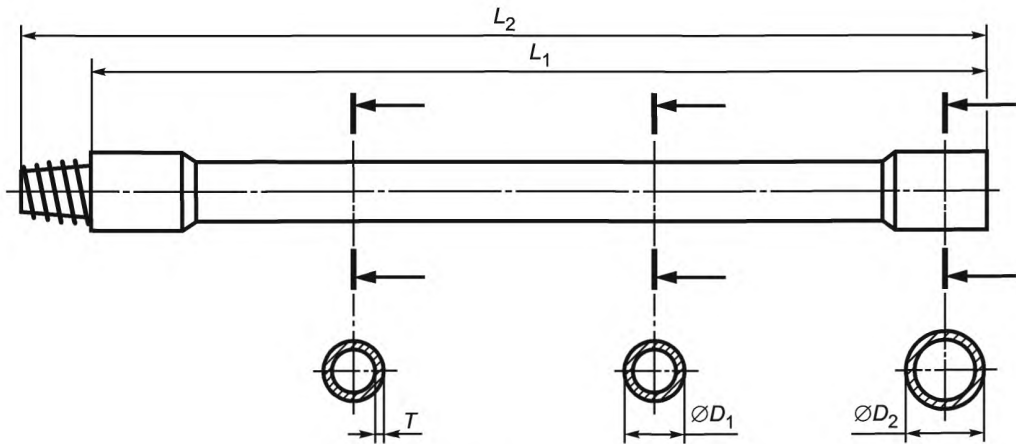
Рисунок 5 — Бурильная труба
