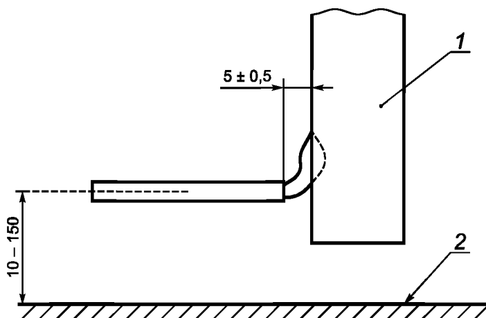
Рисунок 2 — Положение горелки с игольчатым пламенем
