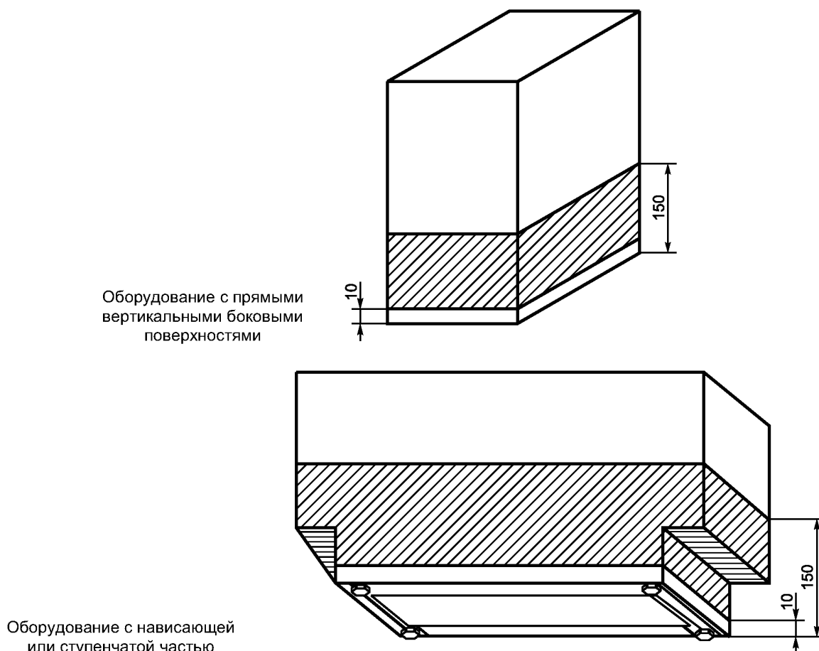
Рисунок 1 — Примеры областей, доступных для пламени свечи
