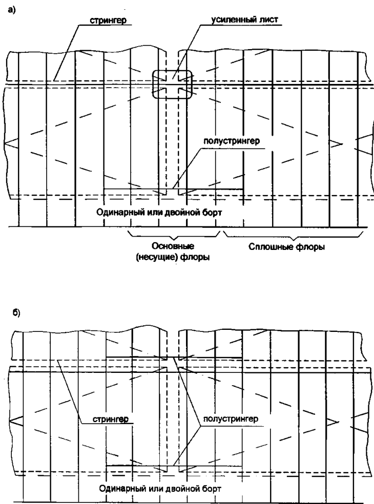
Рис. 3.5.2.2-1 Поперечная система набора
