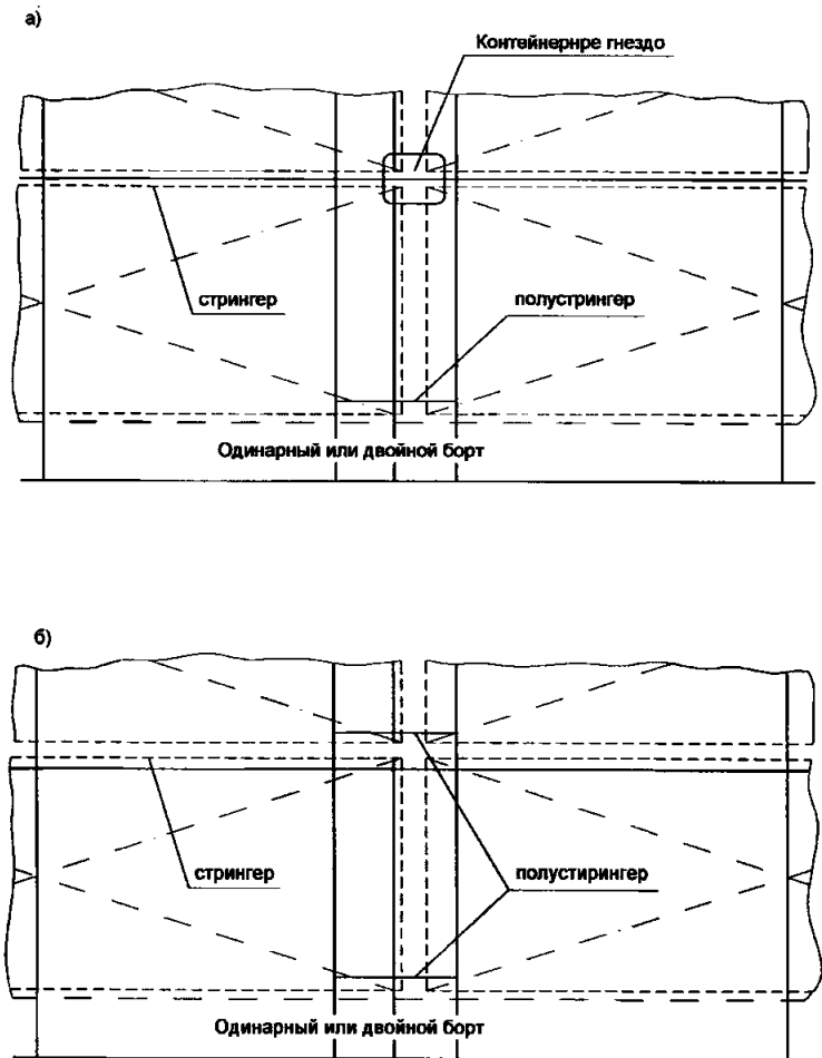
Рис. 3.5.2.2-2 Продольная система набора
