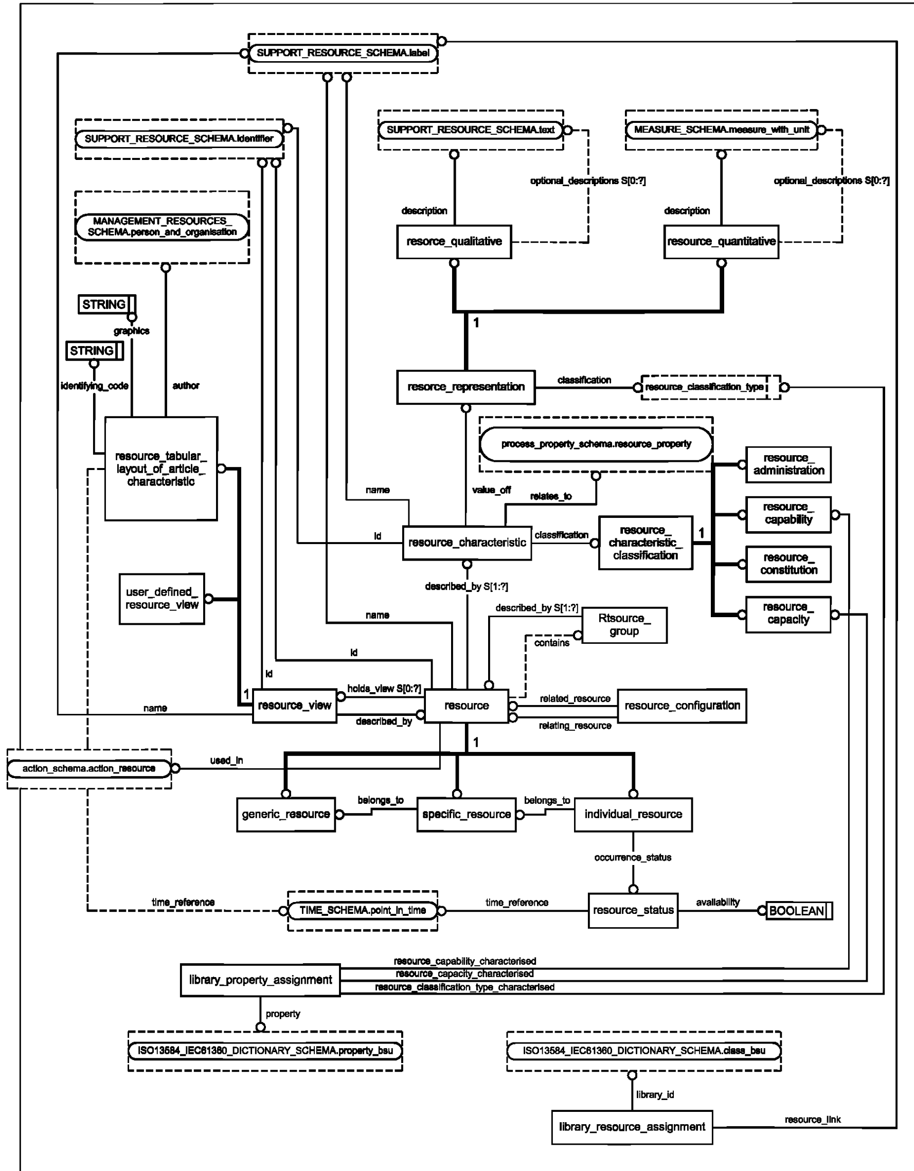
Рисунок D.1 — Схема Resources_usage_management — схема EXPRESS-G
