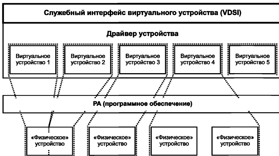
Рисунок 3 — Отображение в памяти виртуальных устройств
