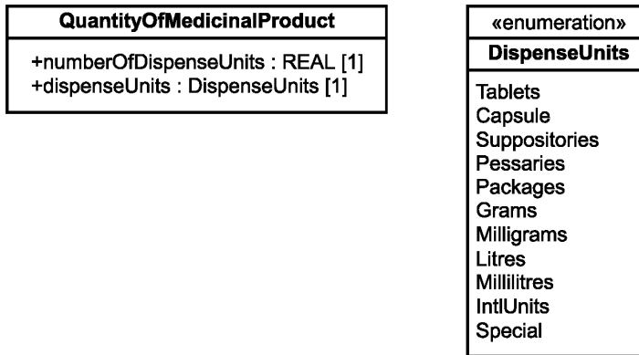
Рисунок 11 — Структура класса «QuantityOfMedicinalProduct»
