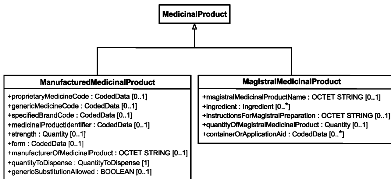
Рисунок 9 — Структура класса «MedicinalProduct»
