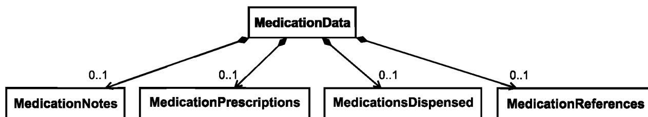
Рисунок 2 — Структура класса «MedicationData»
