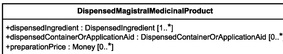
Рисунок 23 — Структура класса «DispensedMagistralMedicinalProduct»
