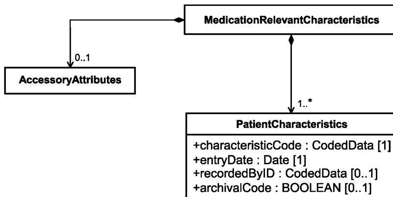
Рисунок 5 — Структура класса «MedicationRelevantCharacteristics»
