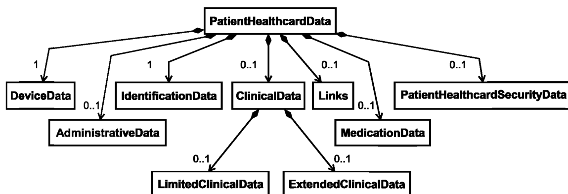
Рисунок 1 — Данные на пластиковой карте пациента. Общая структура
