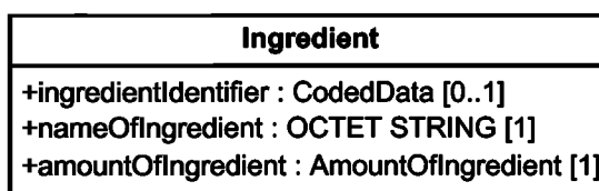
Рисунок 13 — Структура класса «Ingredient»
