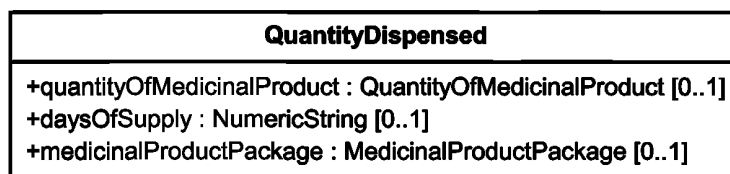
Рисунок 21 — Структура класса «QuantityDispensed»
