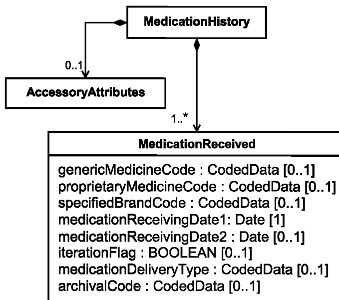
Рисунок 4 — Структура класса «MedicationHistory»
