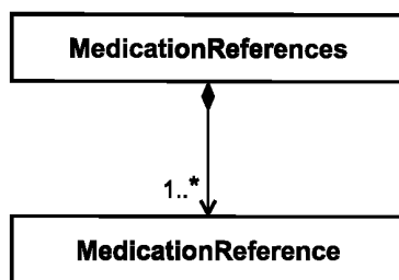
Рисунок 26 — Структура класса «MedicationReferences»
