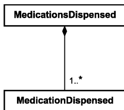
Рисунок 17 — Структура класса «MedicationsDispensed»
