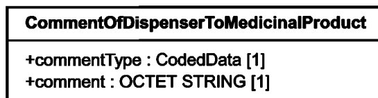
Рисунок 22 — Структура класса «CommentOfDispenserToMedicinalProduct»
