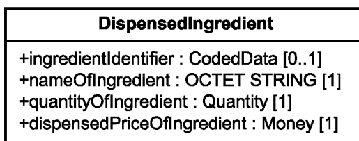
Рисунок 24 — Структура класса «DispensedIngredient»
