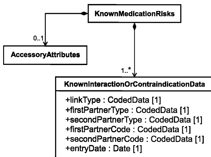
Рисунок 6 — Структура класса «KnownMedicationRisks»
