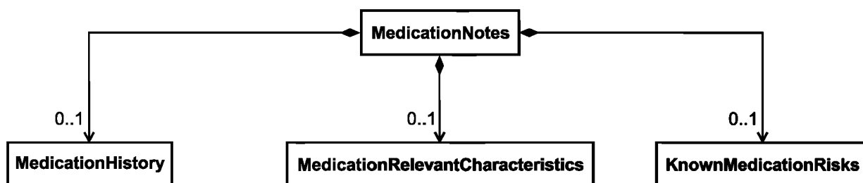
Рисунок 3 — Структура класса «MedicationNotes»
