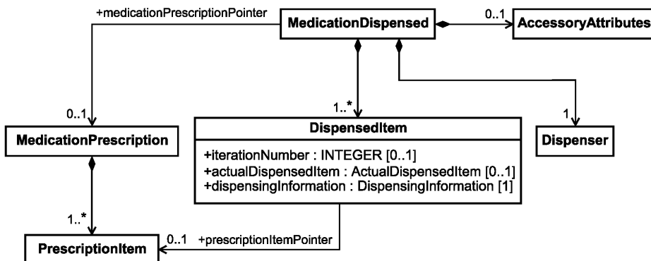
Рисунок 18 — Структура класса «MedicationDispensed»
