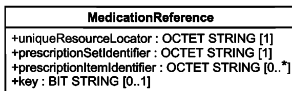
Рисунок 27 — Структура класса «MedicationReference»
