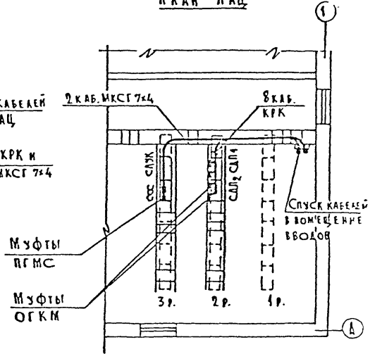
Разрез 1-1
