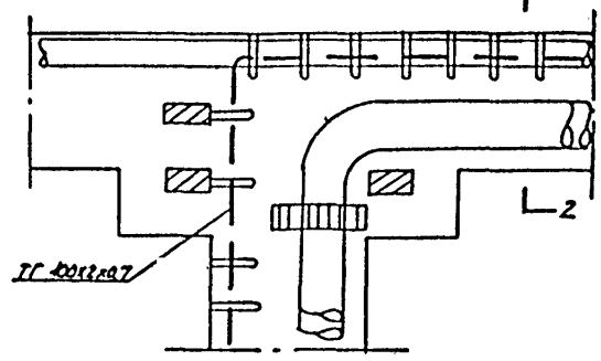
План узла 30 № 25
