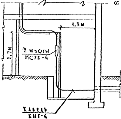
Разрез 2-2
