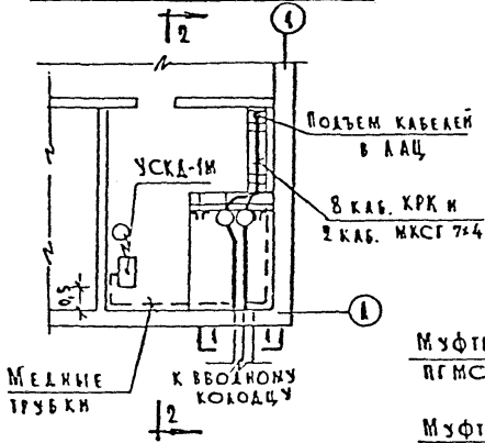
План помещения вводов кабелей
