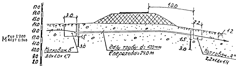
Профиль
