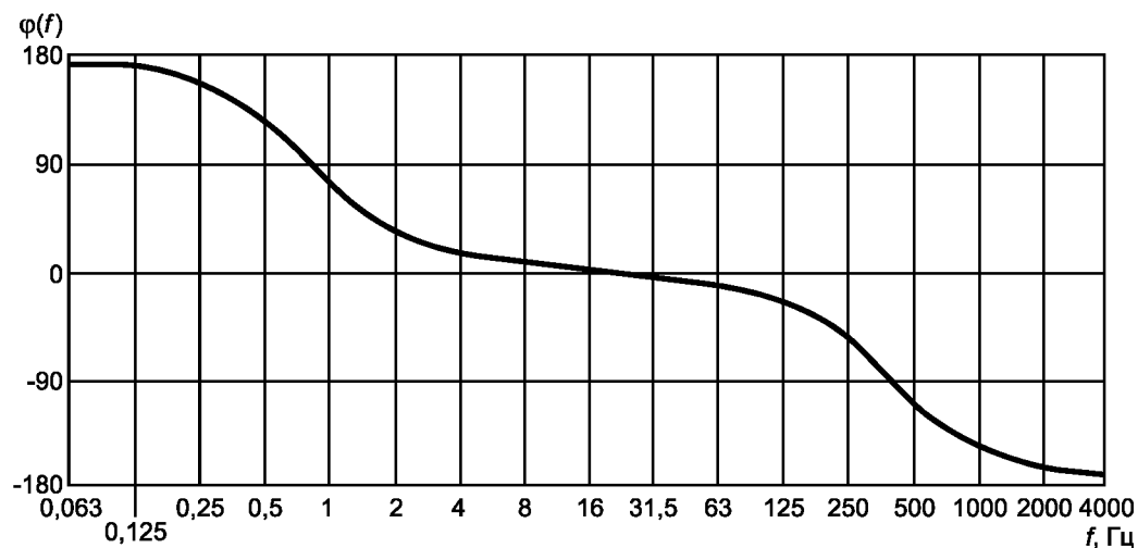
Рисунок 3 — Фазочастотная характеристика измерительной цепи
