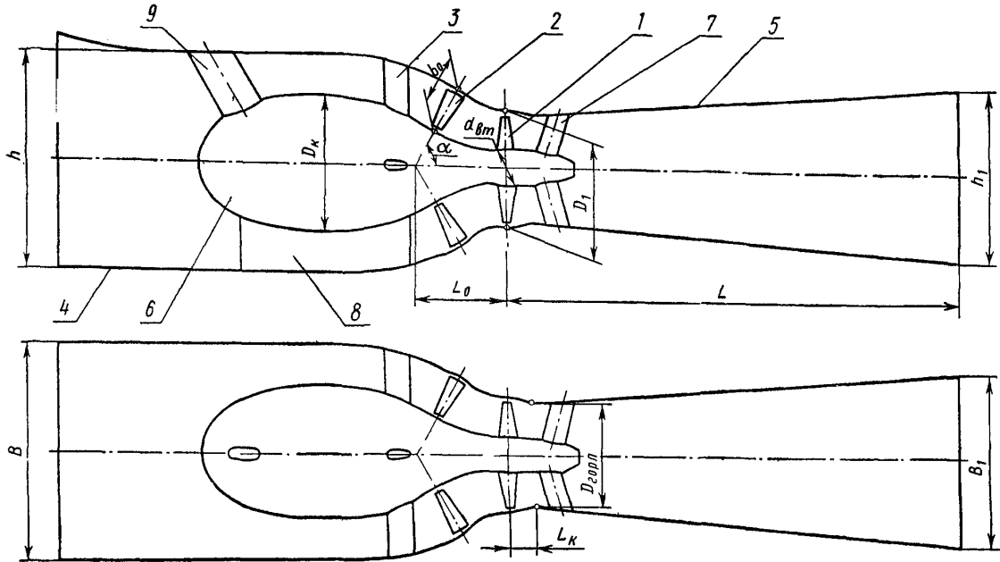
1 — колесо рабочее; 2 — аппарат направляющий; 3 — статор; 4 — камера подводящая; 5 — труба отсасывающая; 6 — капсула; 7 — статор выходной; 8 — бычок опорный; 9 — колонна проходная
