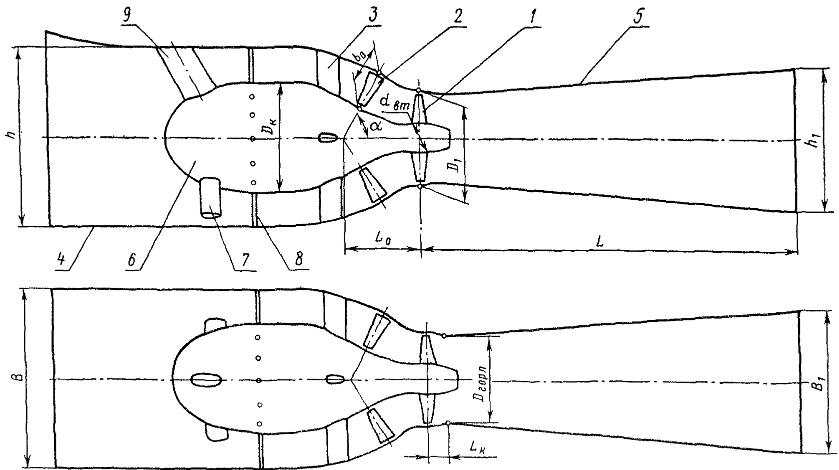
1 — колесо рабочее; 2 — аппарат направляющий; 3 — статор; 4 — камера подводящая; 5 — труба отсасывающая; 6 — капсула; 7 — колонна распорная; 8 — растяжка; 9 — колонна проходная
