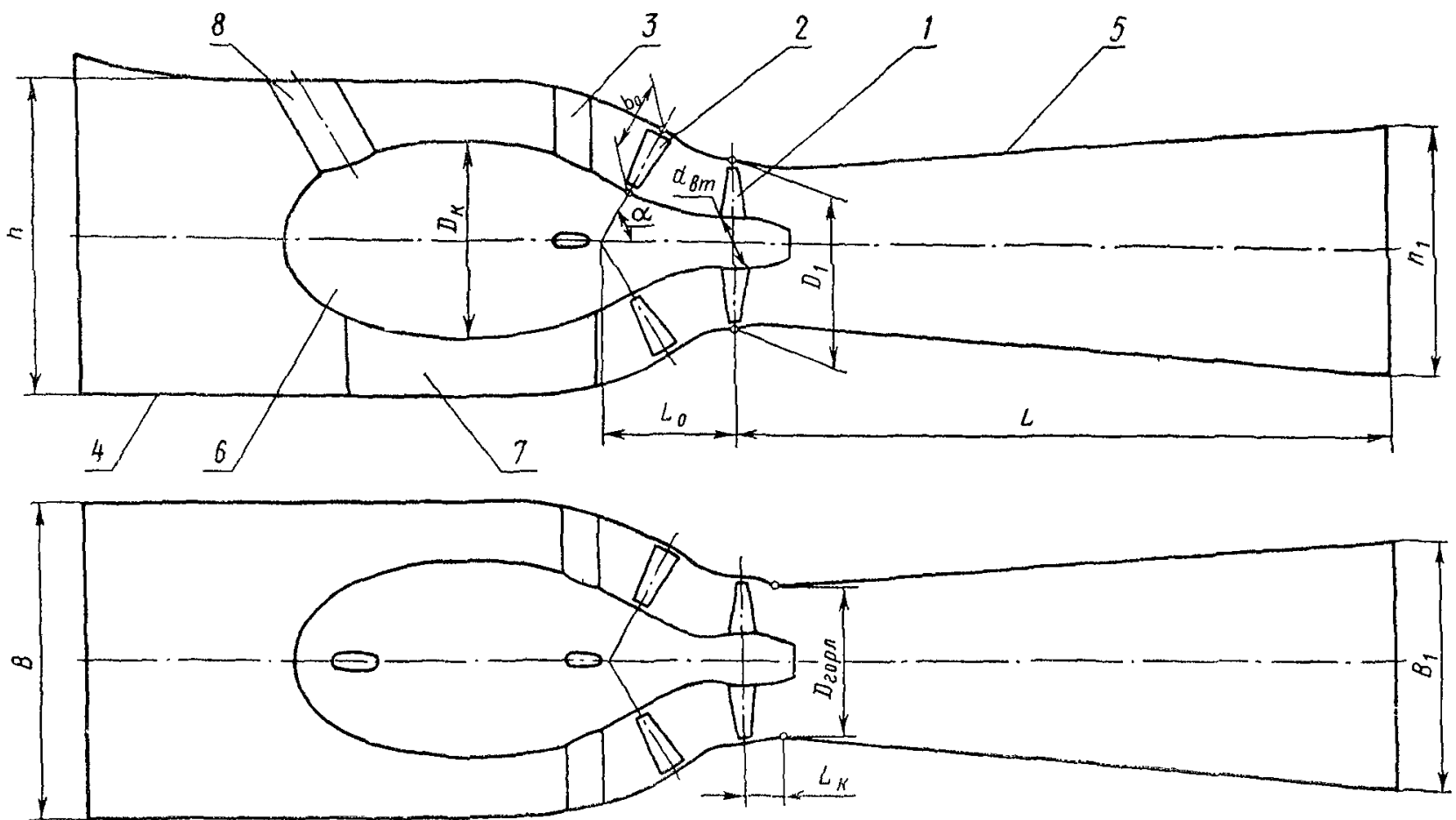
1 — колесо рабочее; 2 — аппарат направляющий; 3 — статор; 4 — камера подводящая; 5 — труба отсасывающая; 6 — капсула; 7 — бычок опорный; 8 — колонна проходная
