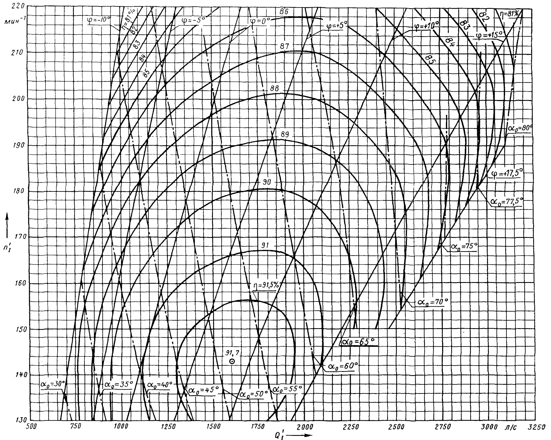
Испытания проведены при напоре гидротурбины от 2,5 до 3 м и температуре 18°C Черт. 20
