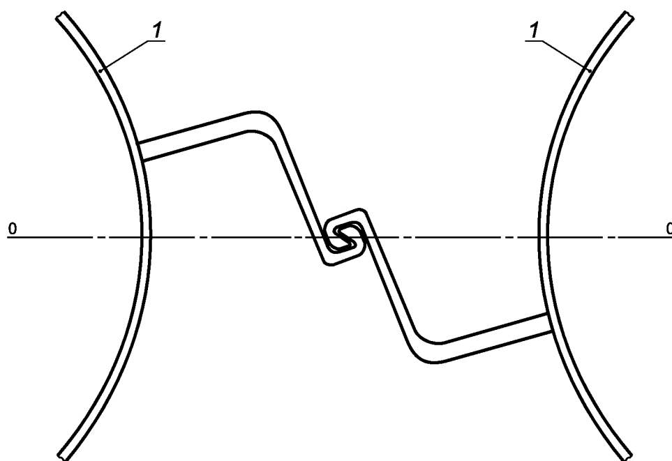
Рисунок 3 — Замковое соединение из раскроя шпунта корытного профиля
