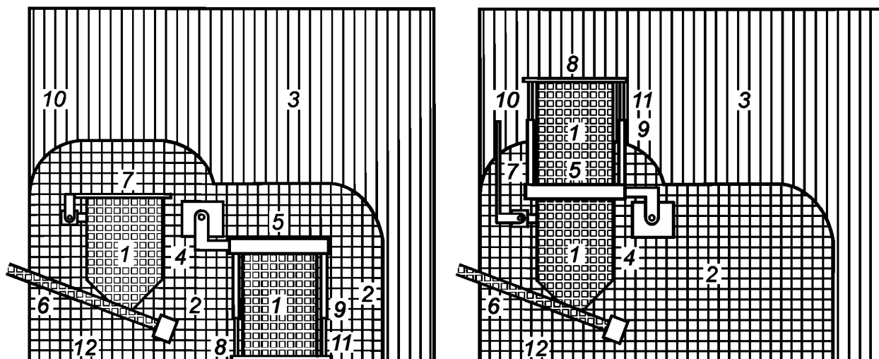
1 — зона класса 20, см. 6.3.2; 2 — зона класса 21, см. 6.3.3; 3 — зона класса 22, см. 6.3.4; 4 — загрузочная воронка; 5 — мембранный клапан; 6 — винтовой конвейер; 7 — люк загрузочной воронки; 8 — барабанная платформа; 9 — гидравлические цилиндры; 10 — стена; 11 — барабан; 12 — основание
