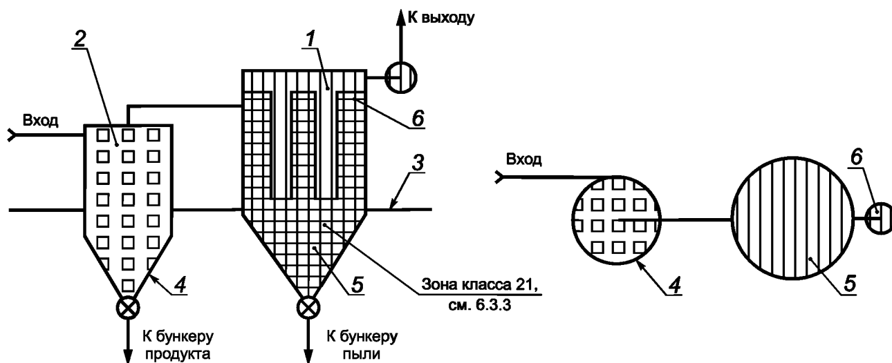
1 — зона класса 22, см. 6.3.4; 2 — зона класса 20, см. 6.3.2; 3 — основание; 4 — циклон; 5 — фильтр; 6 — удаляющий вентилятор
