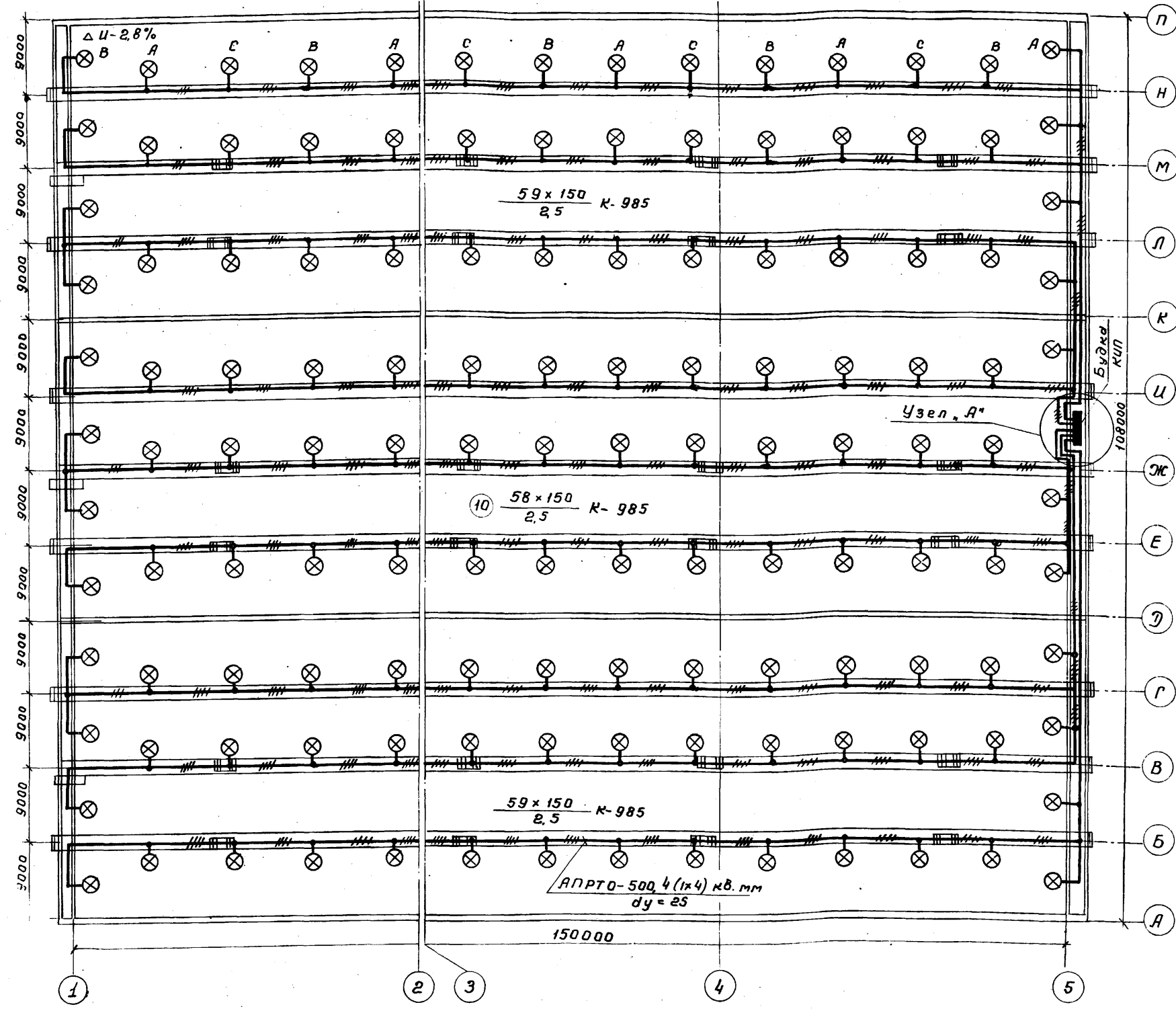
План м 1:400
