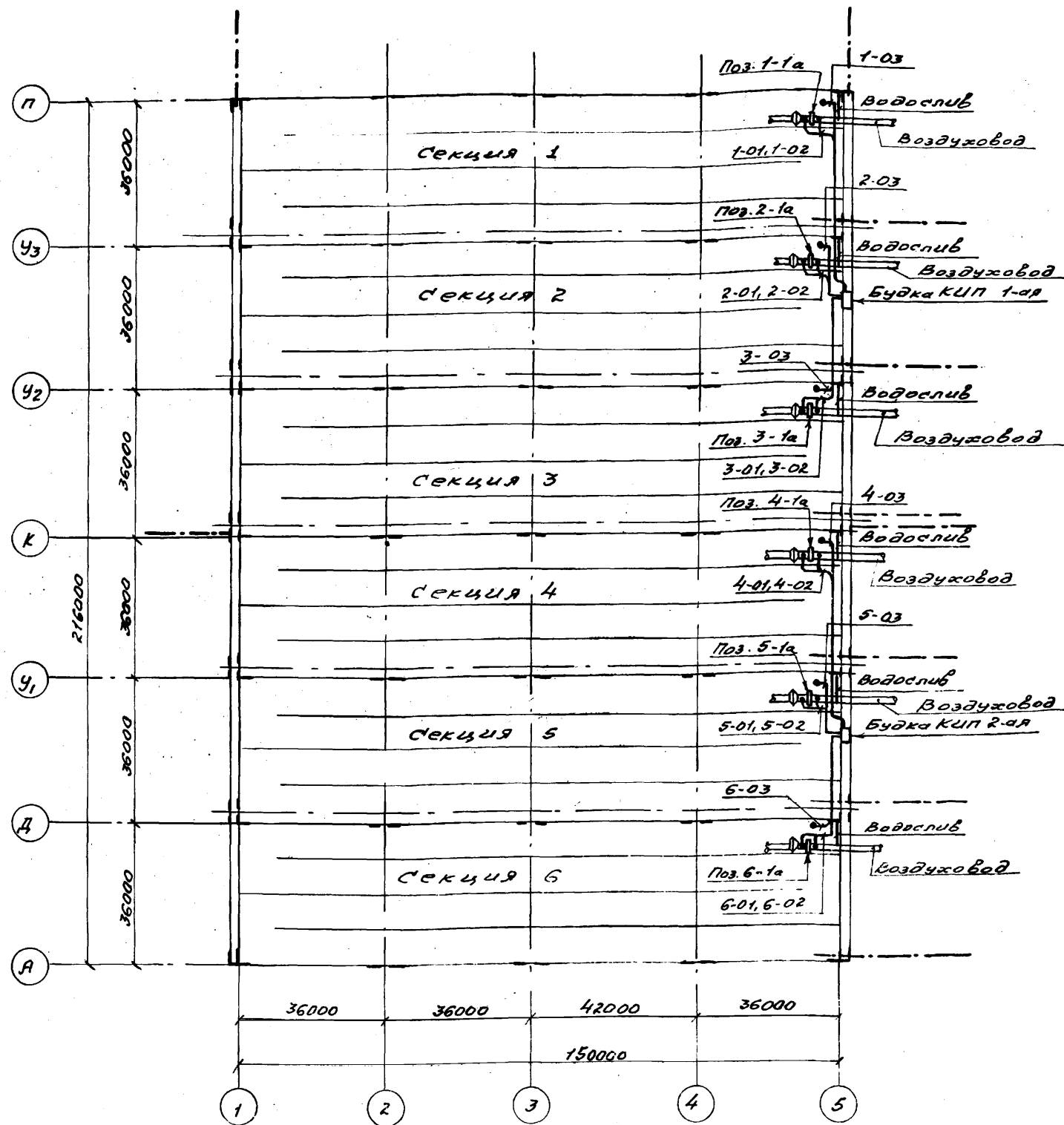
План шестисекционного аэротенка
