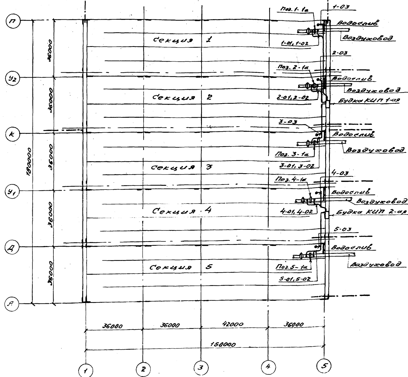
План пятисекционного аэротенка
