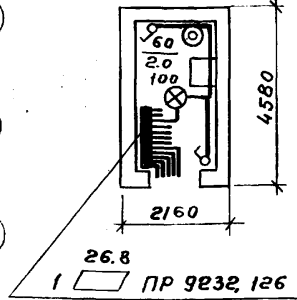
Узел "А" План будки КЦП м 1:100
