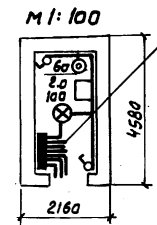
Узел „А“ ПЛАН БУДКИ КИП 1 П45 кВт ПР 9232-126
