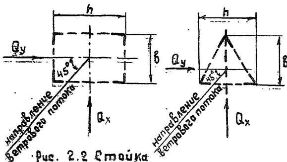
Рис. 2.2 Стойки
