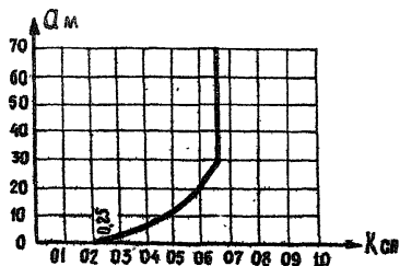
Зависимость коэффициента спада ( K_{cp} ) от длины участка ( a )
