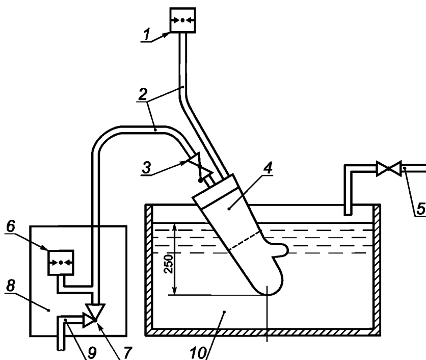
1 — манометр; 2 — гибкие трубки; 3 невозвратный клапан; 4 — круглый удерживающий стержень; 5 — подача воды; 6 — манометр; 7 — регулятор давления; 8 — панель инструментов; 9 — подача сжатого воздуха; 10 — ванна
