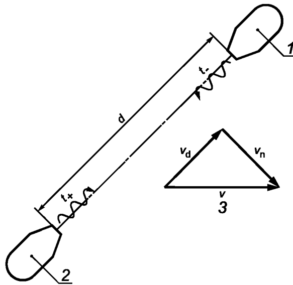
Рисунок В.1 — Принцип работы анемометра
