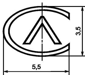
Рисунок А.2 — Сталь с пределом пропорциональности \sigma_0 \geq 700 МПа
