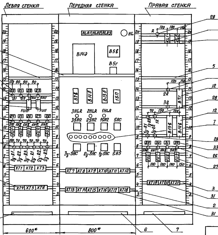
РАЗМЕТКА ЩИТА ПОД КРЕПЛЕНИЕ РП160
