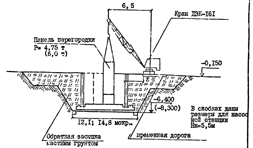
ДЕТАЛЬ УСТРОЙСТВА ДРЕНАЖНОГО ПРИЕМА
