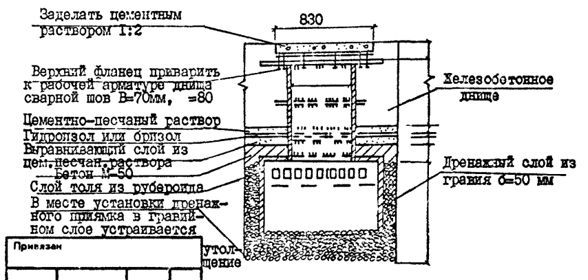
ДЕТАЛЬ УСТРОЙСТВА ДРЕНАЖНОГО ПРИЕМА
