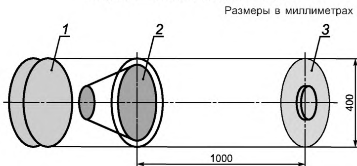
Рисунок 1 — Испытательная установка
