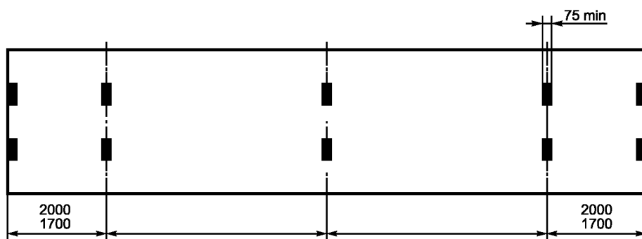
Рисунок Б.3 — Минимальное количество пар опорных (контактных) площадок контейнеров типов 1AAA, 1AA, 1A и 1AX без тоннеля для захвата типа «шея гуся»
