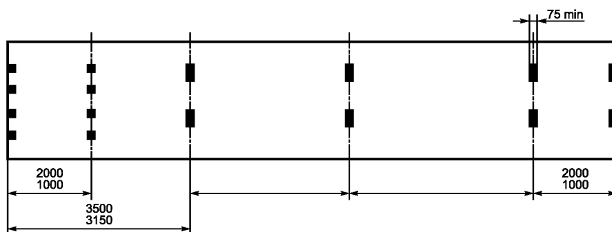
Рисунок Б.4 — Минимальное количество пар опорных (контактных) площадок контейнеров типов 1AAA, 1AA, 1A и 1AX с тоннелем для захвата типа «шея гуся»
