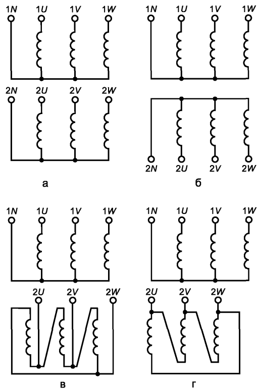
Рисунок Ж.4 — Маркировка трехфазных двухобмоточных трансформаторов
