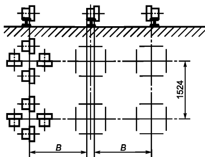
Рисунок Г.2 — Трансформаторы массой от 200 до 255 т
