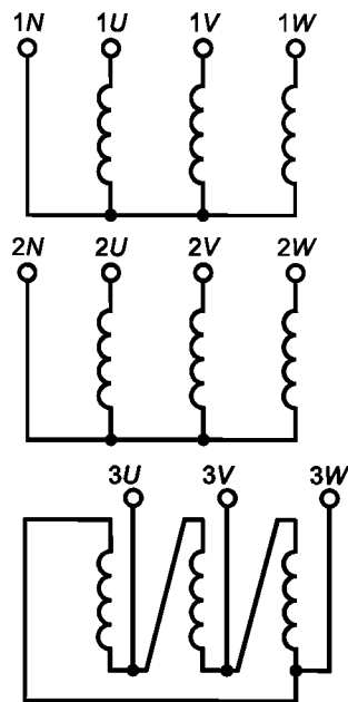
Рисунок Ж.5 — Маркировка трехфазного трехобмоточного трансформатора ( Y_H/Y_H/D-0-5 )
