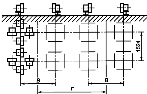
Рисунок Г.3 — Трансформаторы массой от 255 до 300 т
