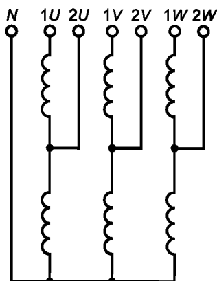
Рисунок Ж.7 — Маркировка трехфазного автотрансформатора ( Y_H\text{авто}/D-0 )
