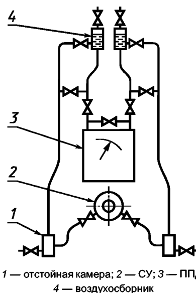
1 — отстойная камера; 2 — СУ; 3 — ППД; 4 — воздухосборник
