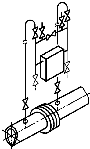
Рисунок Г.1 — ППД над трубо- водом
