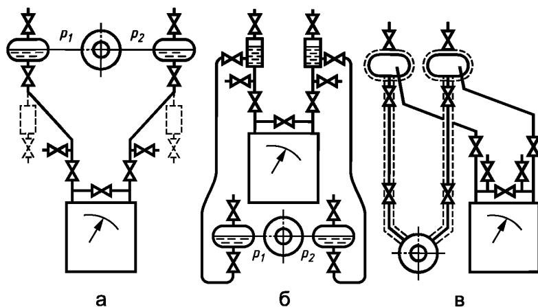
Рисунок 3 — Схемы расположения уравнительных сосудов и соединительных трубок
