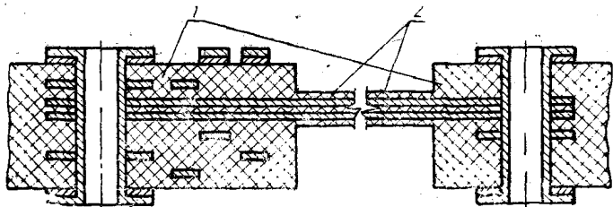
1 — материал основания (жесткая часть); 2 — материал основания (гибкая часть)
