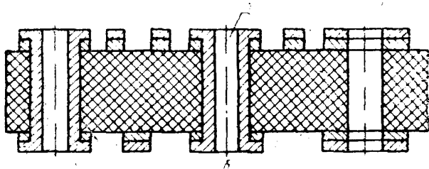
1 — материал основания; 2 — проводящий рисунок; 3 — металлизированное отверстие
