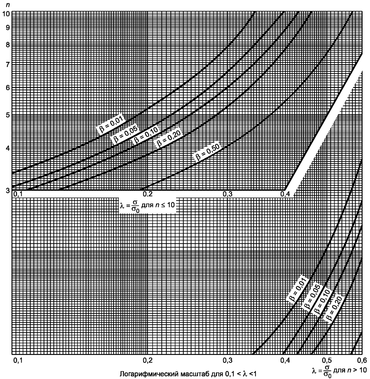
Рисунок 5.2 — Двусторонний критерий сравнения дисперсии с заданным значением (риск первого рода \alpha = 0,05 ), лист 1
