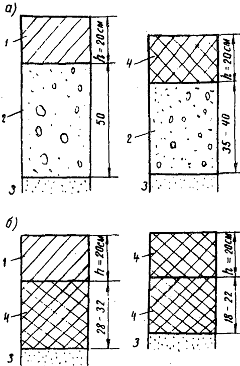
Рис.1. Конструкция оснований и морозозащитных слоев из укрепленных золошлаковых смесей: а-существующая конструкция; б-рекомендуемые; 1-основание из цемента или щебня; 2-морозозащитный слой из песков или крупнообломочных грунтов; 3-земляное полотно; 4-основание или морозозащитный слой из золошлаковых смесей, укрепленных цементом без добавок или с добавками жидкого битума либо СДБ; золой уноса без добавок или с добавками СДБ; гранулированным доменным шлаком с добавками цемента, известью
