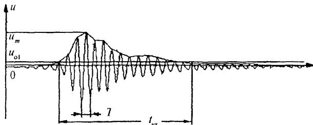
Рис. 1 Типичная импульсная характеристика ПАЭ
