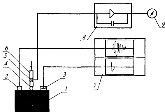
Рис. 2. Схема измерения 1:
