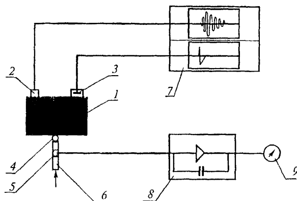
Рис. 3. Схема измерения 2:
