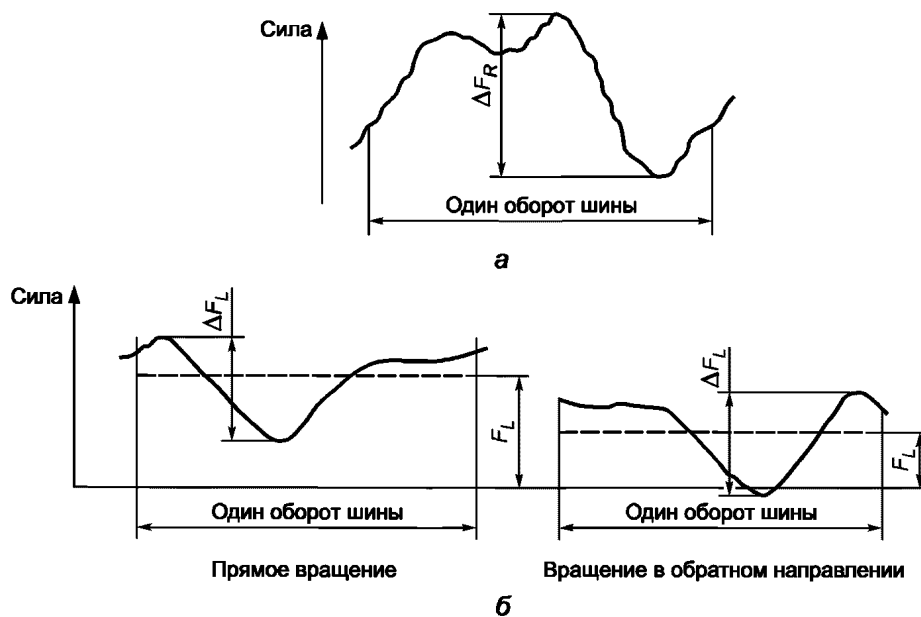
а — радиальная сила; б — боковая сила
