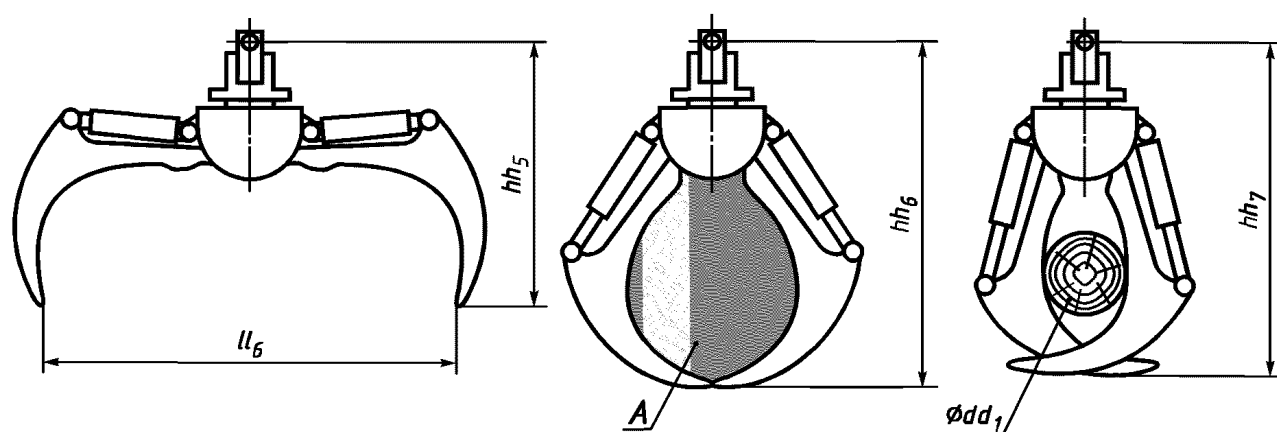
Рисунок 5 — Конструктивные параметры захвата
