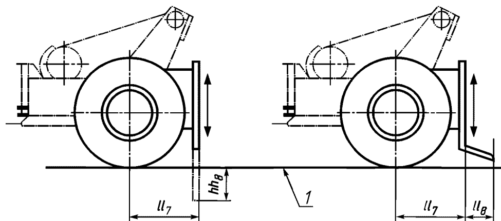
Рисунок 5 — Конструктивные параметры захвата
