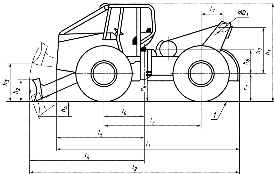
Рисунок 1 — Машина трелевочная чокерная колесная с шарнирно-сочлененной рамой
