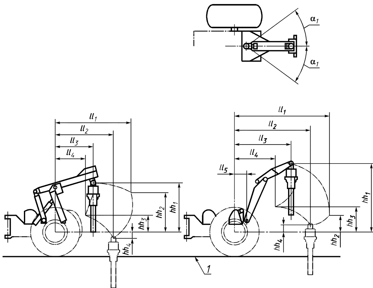
Рисунок 4 — Стрела с захватом
