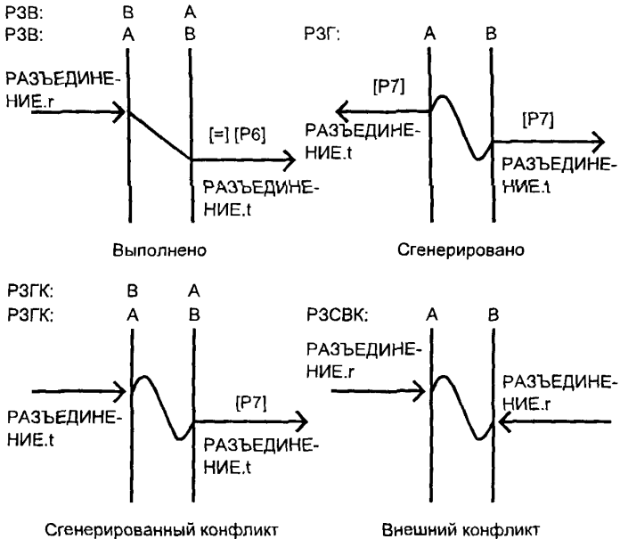
Рисунок 9 — Фаза «разъединение ССУ»
