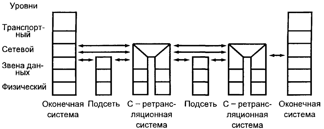
А – Полная архитектурная модель (ИСО 8648)
