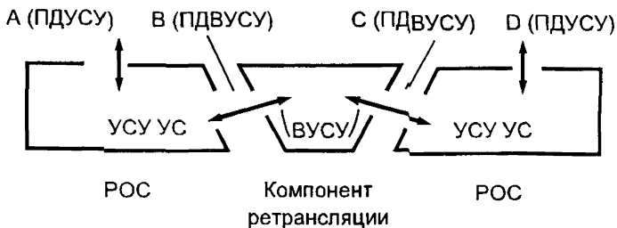
Рисунок С.2 — Модель ретрансляции на сетевом уровне
