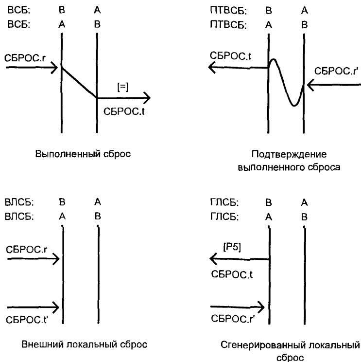
Рисунок 8 — Передача данных, подфаза «сброс»
