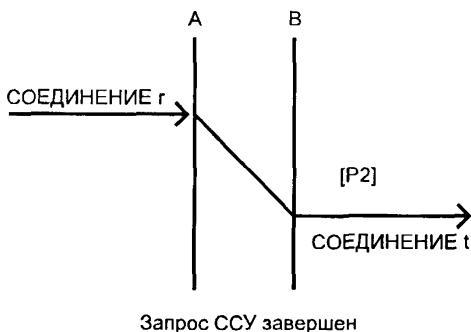
Рисунок 4 — Установление ССУ, подфаза «запрос ССУ»
