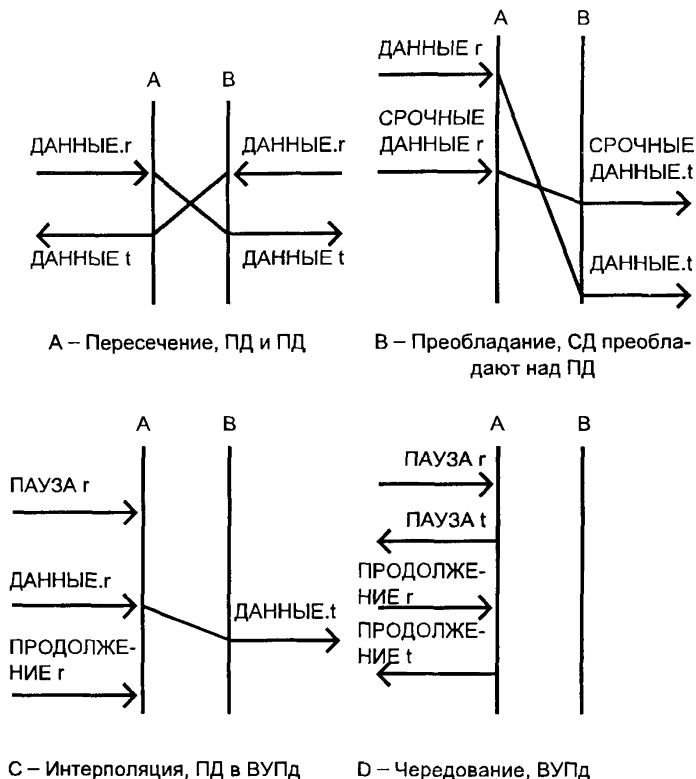
Рисунок 11 — Непрямые комбинации элементарных последовательностей
