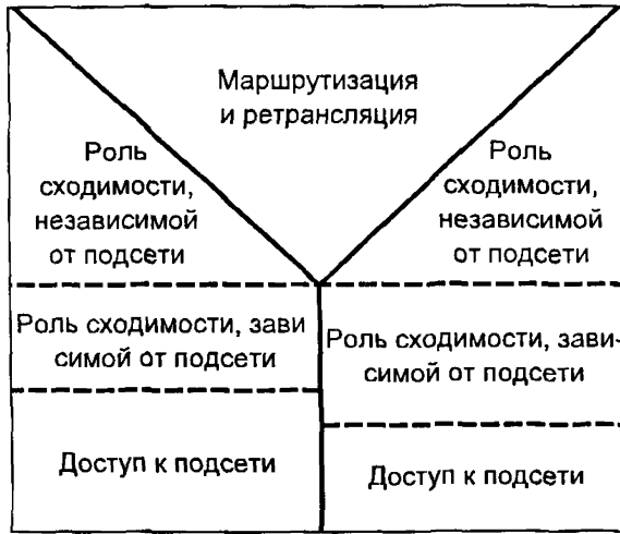
Рисунок В 1 — Внутренняя структура функций S-логического объекта ретрансляции
