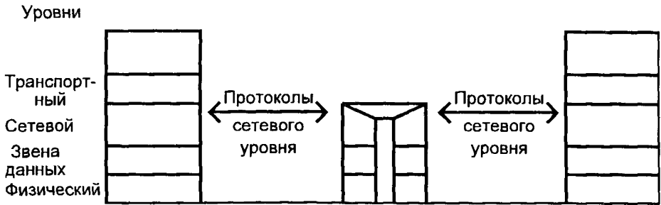
А — Представление ИСО 8648 с ретрансляционной моделью
