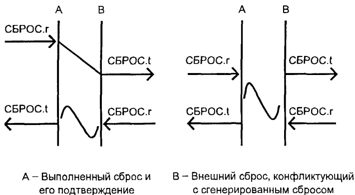
Рисунок 13 — Примеры базового сброса
