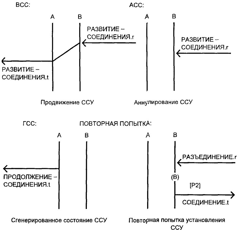
Рисунок 5 — Установление ССУ, подфаза «развитие ССУ»
