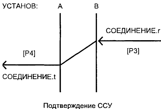
Рисунок 6 — Установление ССУ, подфазы «подтверждение ССУ»
