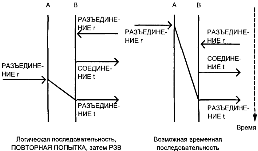
Рисунок 10 — Пример выполнения элементарных последовательностей
