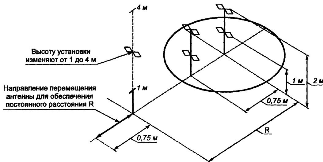
Рисунок Д.4 — Расположения антенн при измерении затухания альтернативной площадки (горизонтальная поляризация) для испытуемого объема с размерами не более 1 \times 1,5 \times 1,5 м и при расстоянии от задней границы объема до ближайшей точки конструкции и/или радиопоглощающего материала более 1 м
