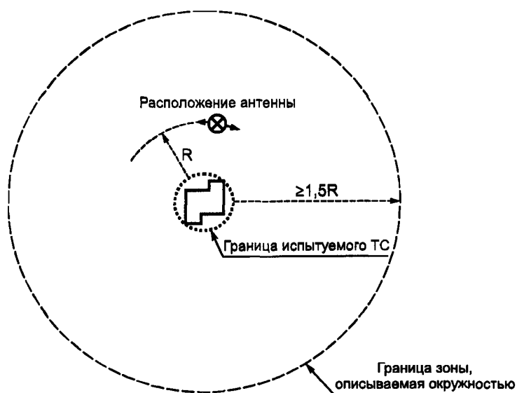
Рисунок В.2 — Зона измерительной площадки со стационарным испытуемым ТС, свободная от предметов, отражающих электромагнитную энергию
