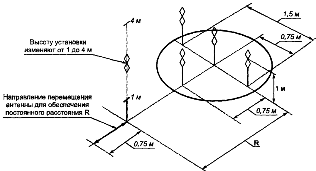
Рисунок Д.3 — Расположения антенн при измерении затухания альтернативной площадки (вертикальная поляризация) для испытуемого объема с размерами не более 1 \times 1,5 \times 1,5 м и при расстоянии от задней границы объема до ближайшей точки конструкции и/или радиопоглощающего материала более 1 м
