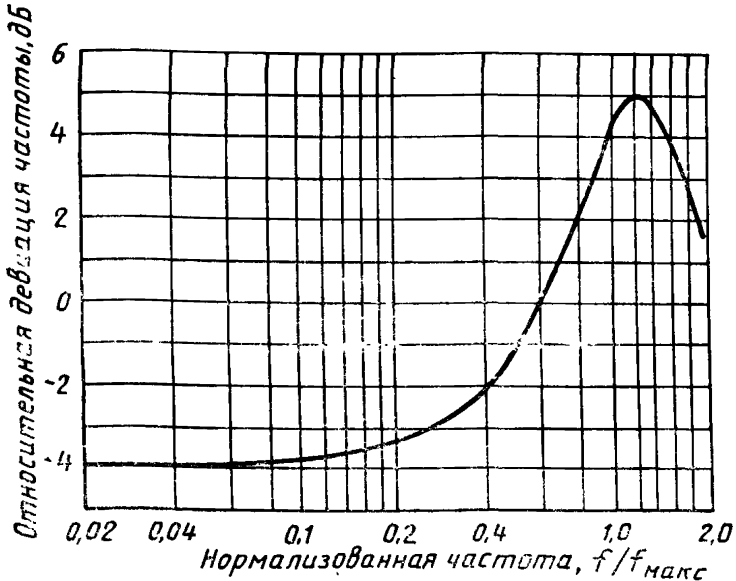
Рисунок В.1 — Характеристика предискажений для телефонии
