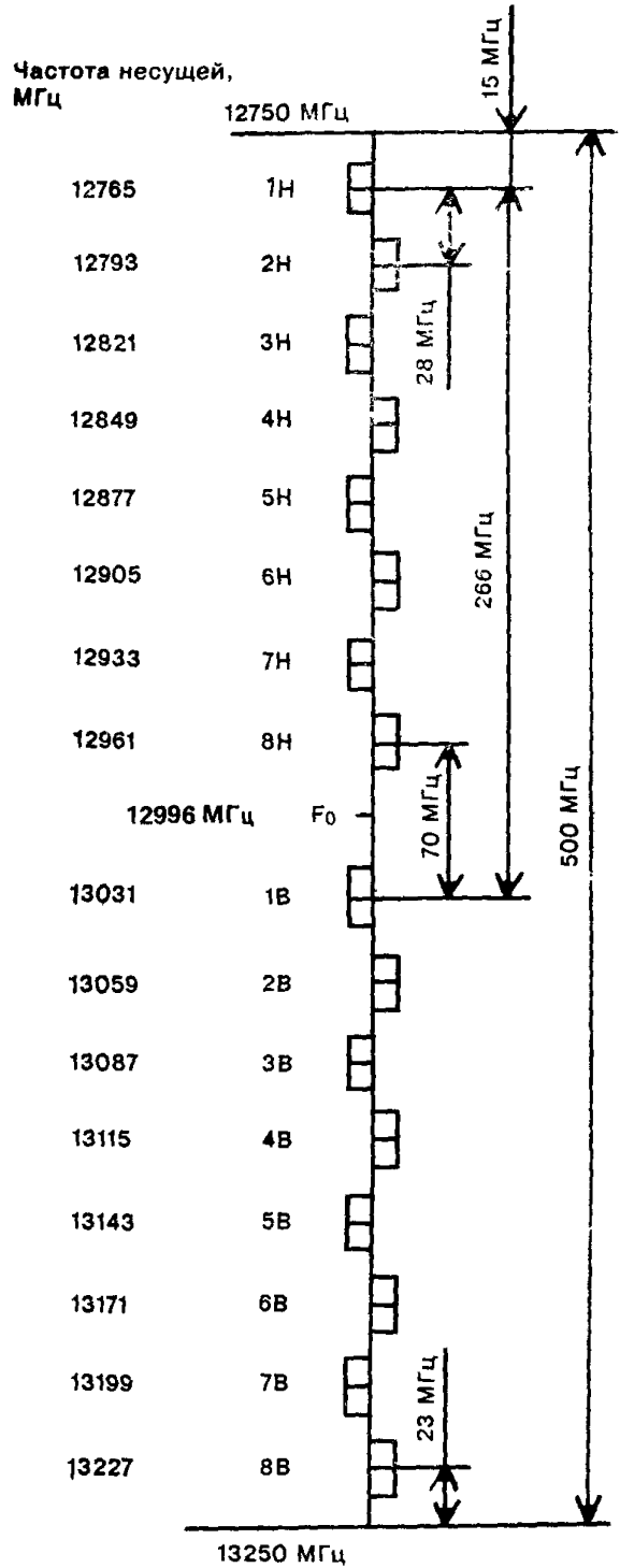
Рисунок Б.8 — Частотный план радиорелейной системы, работающей в диапазоне 13 ГГц
