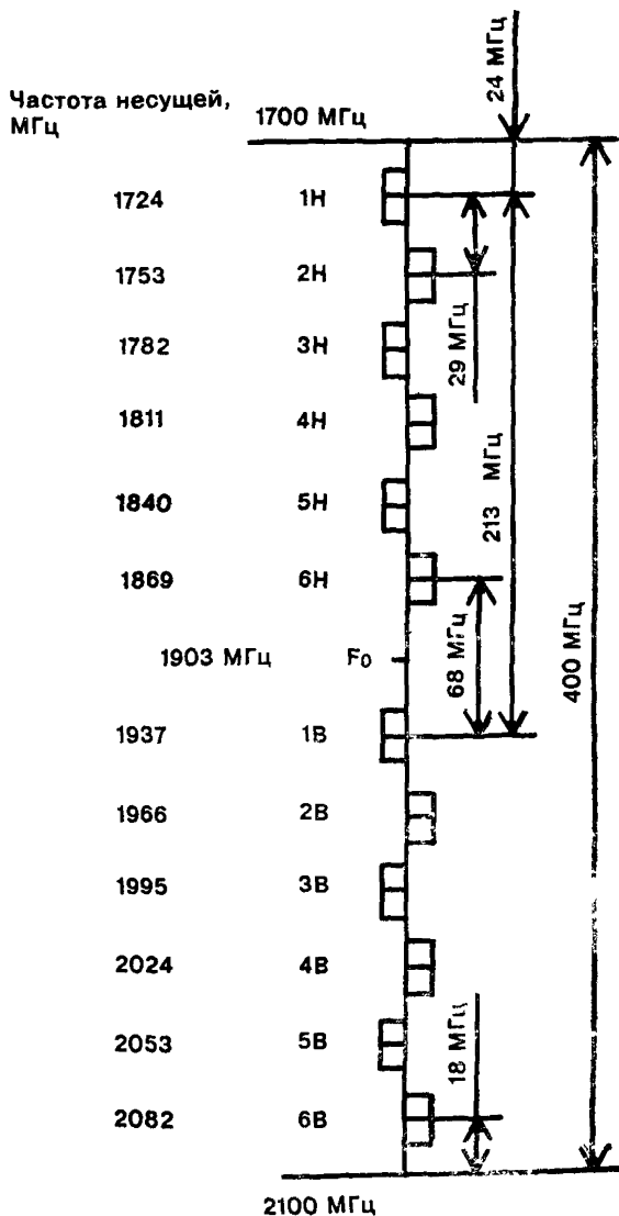
Рисунок Б.3 — Частотный план радиорелейной системы, работающей в диапазоне 2 ГГц
