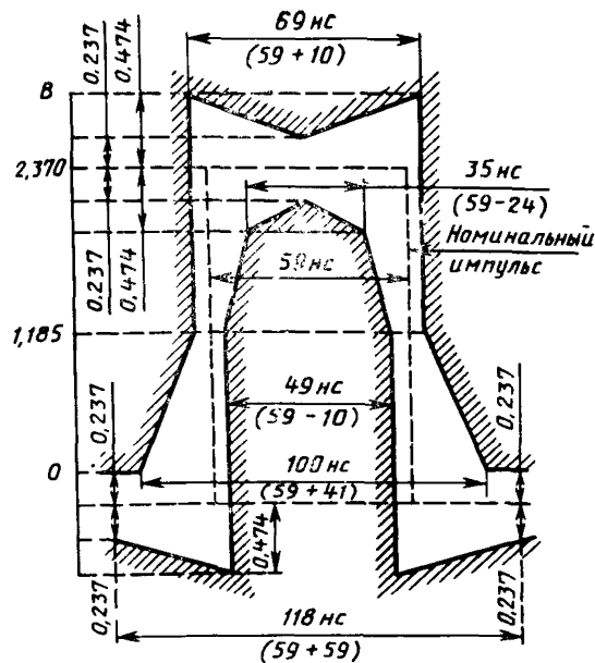
Рисунок 5 — Маска импульса на стыке на 8,448 Мбит/с.
