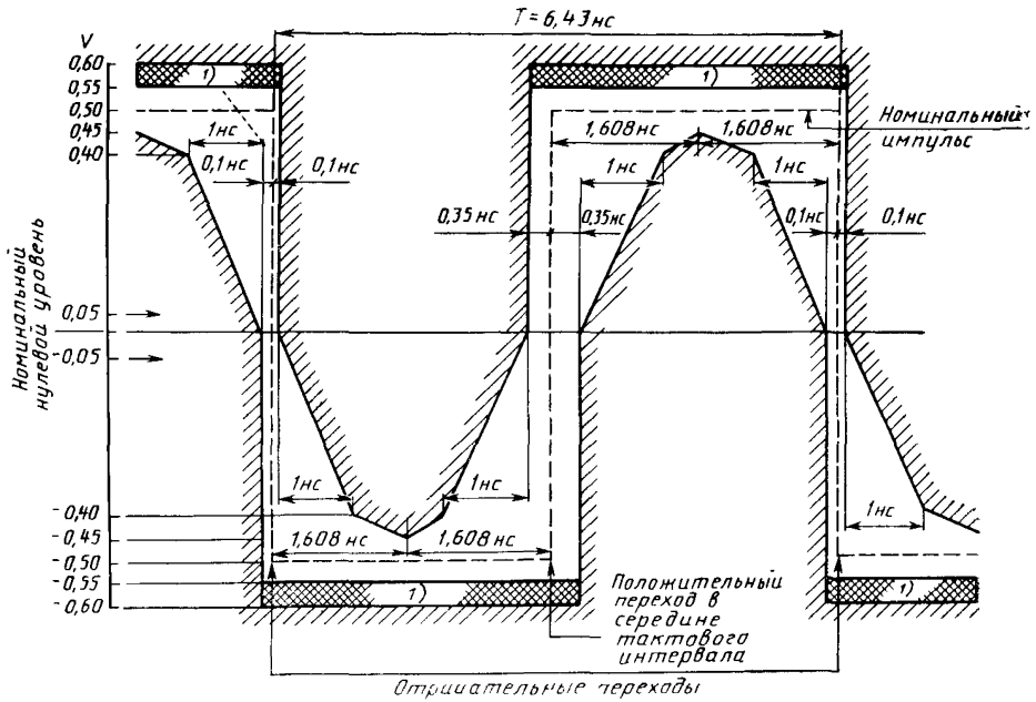
Рисунок 9 — Маска импульса, соответствующая 0, на стыке на 155,520 Мбит/с
