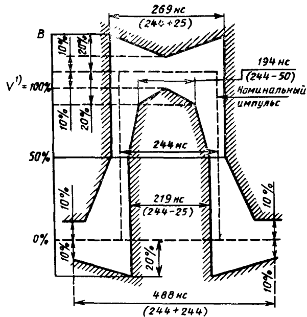
Рисунок 4 — Маска импульса на стыке на 2,048 Мбит/с
