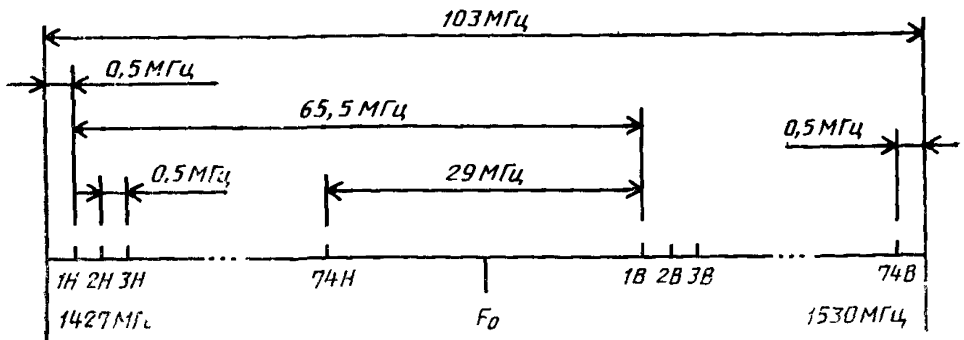
Рисунок Б.2 — Частотный план радиорелейной системы, работающей в диапазоне 1427—1530 МГц
