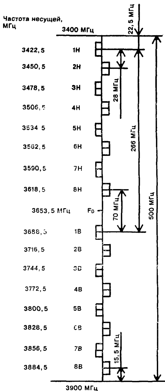
Рисунок Б.5 — Частотный план радиорелейной системы, работающей в диапазоне 4 ГГц
