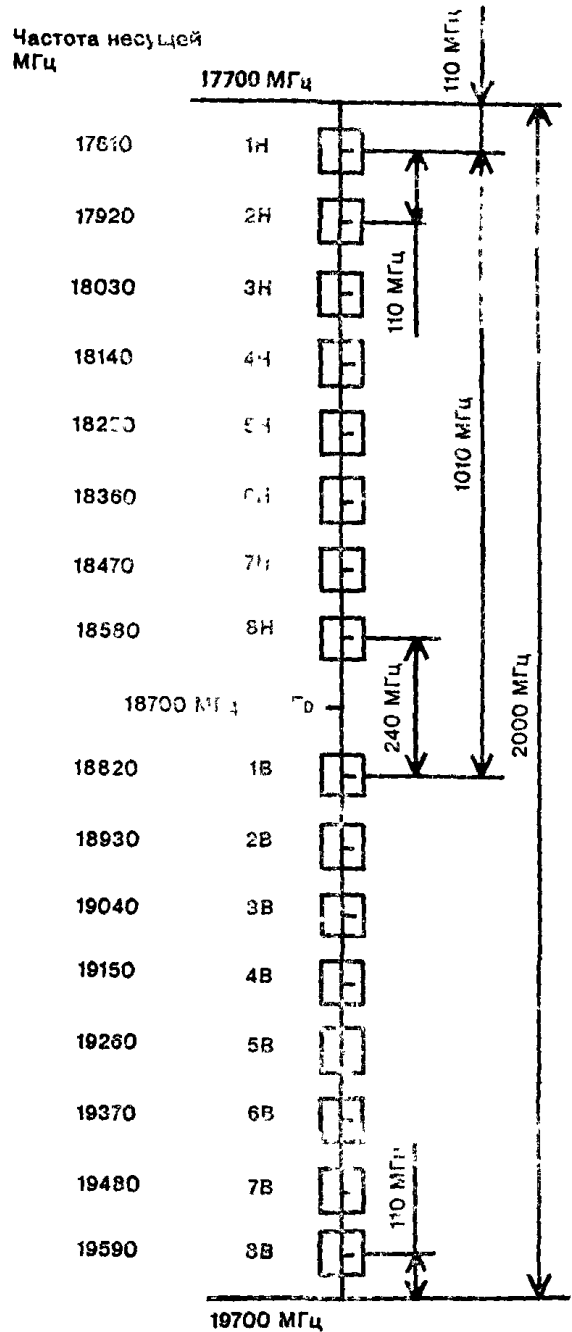
Рисунок Б.13 — Частотный план радиорелейной системы, работающей в диапазоне 17,7—19,7 ГГц (при совпадающих частотах радиостволлов)
