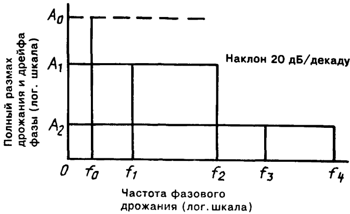
Рисунок 11 — Шаблон максимального допустимого входного фазового дрожания и дрейфа фазы для аппаратуры радиорелейных систем псевдохронной цифровой иерархии
