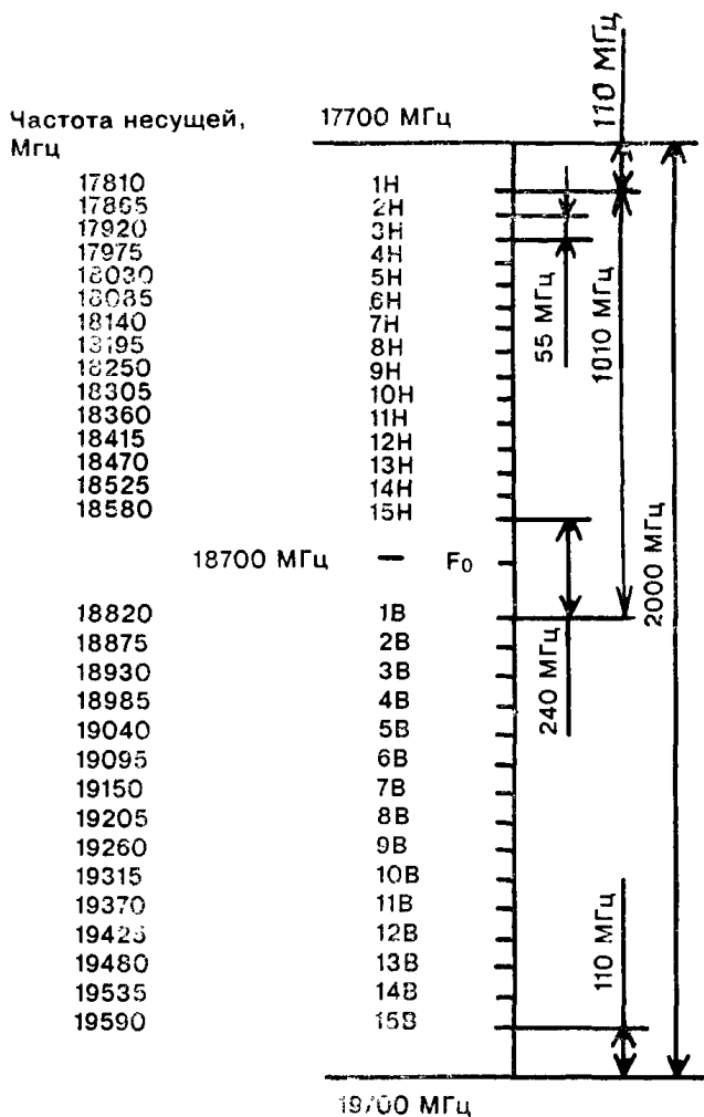
Рисунок Б.14 — Частотный план радиорелейной системы, работающей в диапазоне 17,7—19,7 ГГц (при чередующихся частотах радиостолбов)
