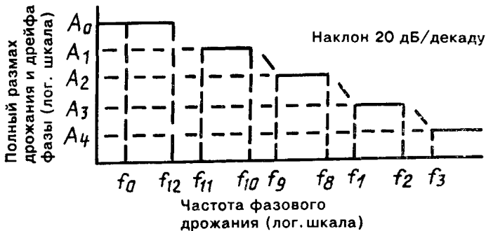
Рисунок 12 — Шаблон максимального допустимого входного фазового дрожания и дрейфа фазы для аппаратуры радиорелейных систем синхронной цифровой иерархии
