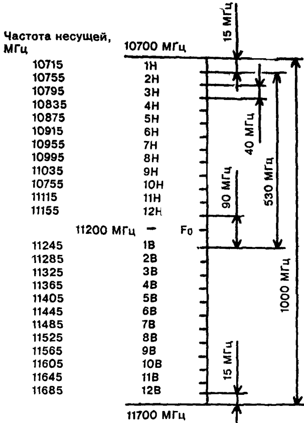
Рисунок Б.11 — Частотный план радиорелейной системы, работающей в диапазоне 11 ГГц
