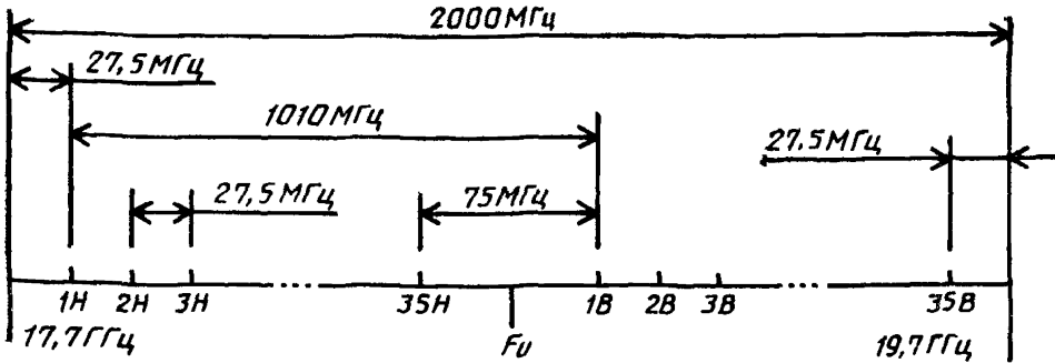
Рисунок Б.15 — Частотный план радиорелейной системы, работающей в диапазоне 17,7–19,7 ГГц (при совпадающих частотах радиостолов)
