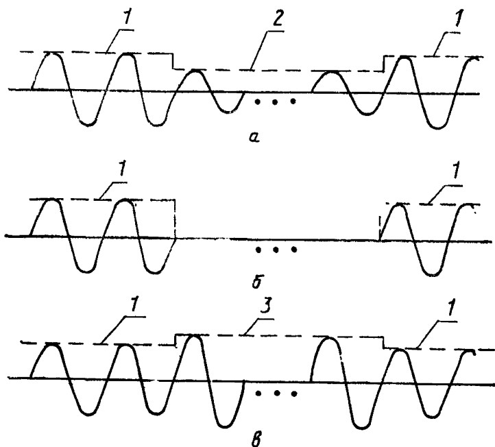
а — провал напряжения; б — прерывание напряжения; в — выброс напряжения; 1 — номинальное напряжение; 2 — пониженное напряжение; 3 — повышенное напряжение
