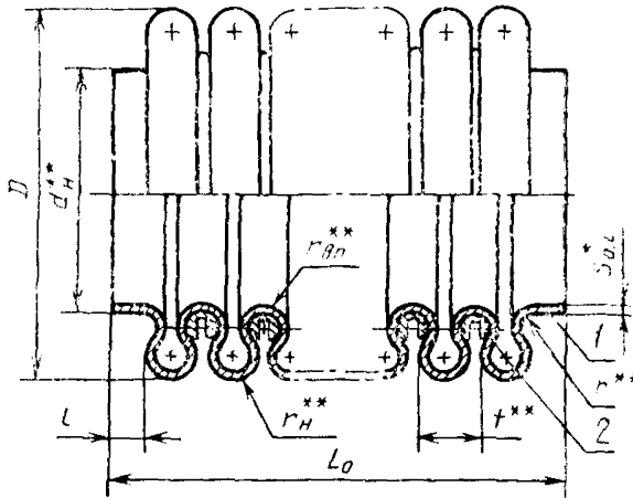
Рисунок 2 — Сильфон, тип 2
