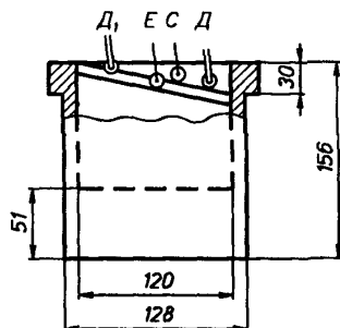
Рисунок 1 — Зональный пробоотборник
