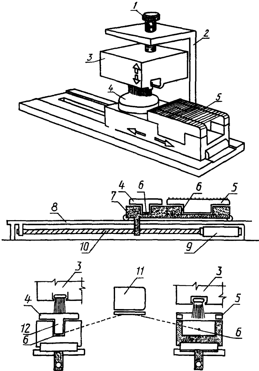
1 — регулировочный винт; 2 — компаратор; 3 — блок; 4 — пластина; 5 — решетка; 6 — датчик силы; 7 — каретка; 8 — салазки; 9 — двигатель; 10 — система винт-гайка; 11 — регистрирующее устрой- ство; 12 — система управления
