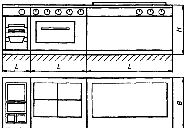
L = 500, 900, 1000, 1500 мм; B = 900 мм; H — в соответствии с 3.3.
