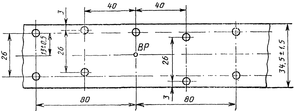
Рисунок 7 — Соединительная деталь
