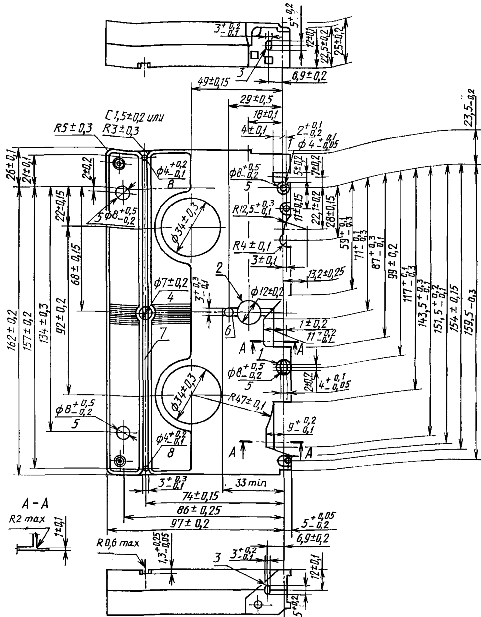
1 — базовое отверстие; 2, 3 — отверстия для прохождения света сенсорного датчика; 4 — отверстие для освобождения тормоза катушки; 5 — опорные поверхности. Отклонение от плоскостности опорных поверхностей не должно быть более 0,2 мм; 6, 7 — направляющий паз для предотвращения неправильной установки видеокассеты в видеомагнитофон; 8 — положение вспомогательного отверстия
