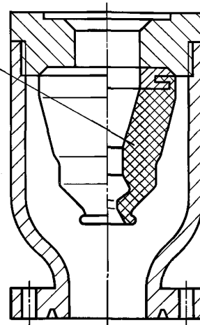
Безотводный устьевой герметизатор (22)
