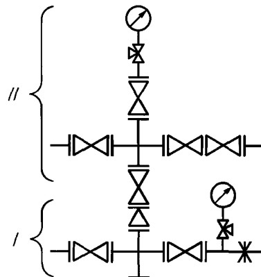
Крестовая одноствольная нагнетательная арматура (26, 31, 36)
