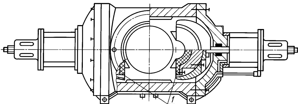
1 — управляемый контактный уплотнитель (плашки) (84, 88)
