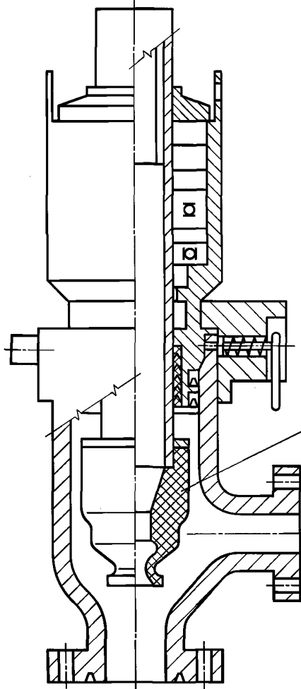
Роторный устьевой герметизатор (23)
