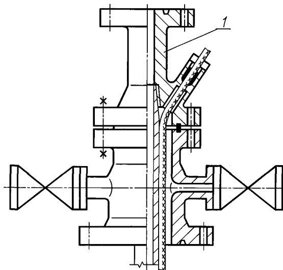
1 — катушка-трубодержатель (73)
