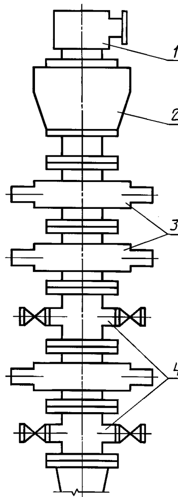
Превенторный блок (12)
