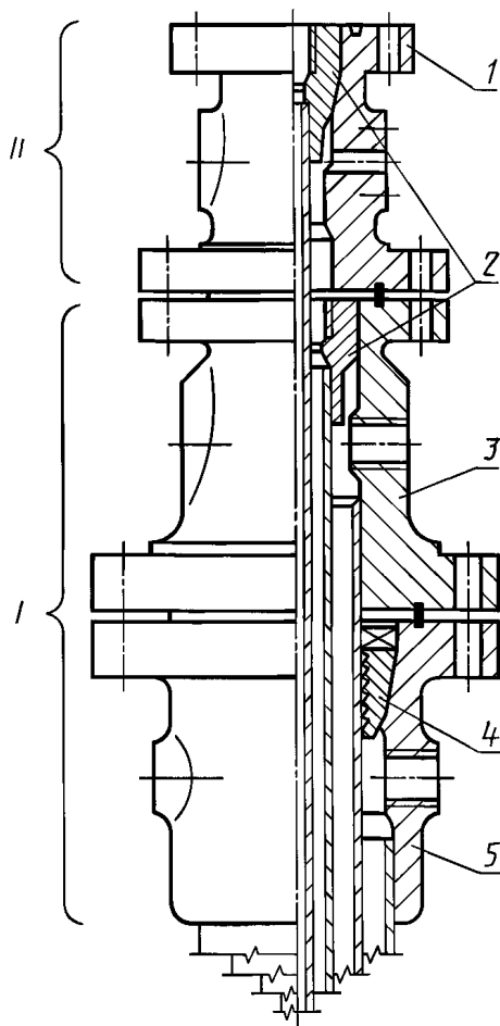
Устьевая обвязка (2)
