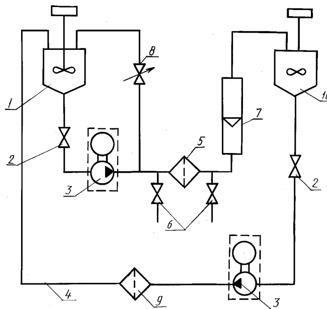
Схема установки для определения полноты отсева фильтрации
