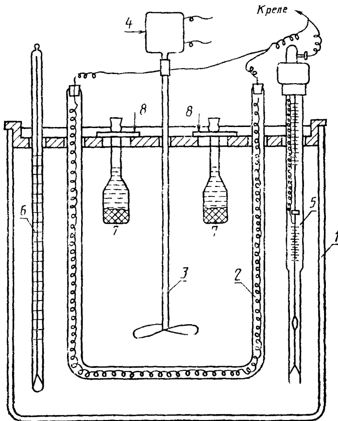
Термостат водяной для определения плотности глинозема
