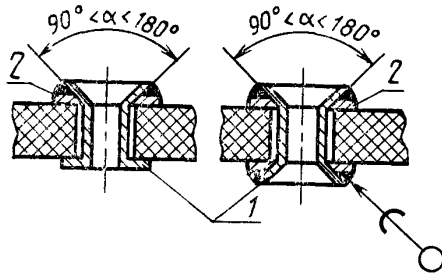
1 — арматура перехода; 2 — контактная площадка
