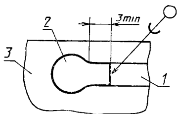
1 — печатный проводник; 2 — новая контактная площадка; 3 — материал основания
