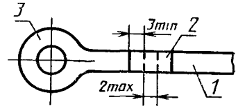
1 — поврежденный печатный проводник; 2 — перемычка; 3 — контактная площадка
