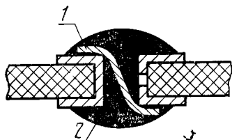
1 — перемычка; 2 — припой
