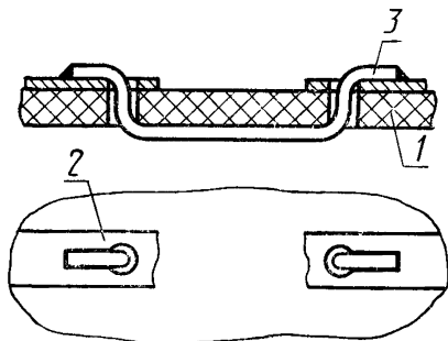
1 — материал основания; 2 — поврежденный печатный проводник; 3 — перемычка
