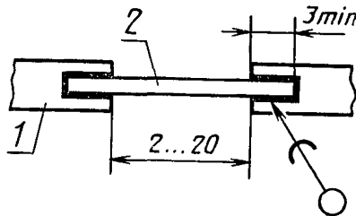
1 — поврежденный печатный проводник; 2 — перемычка
