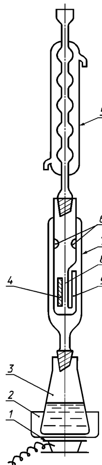
Установка для проведения горячей экстракции полимера
