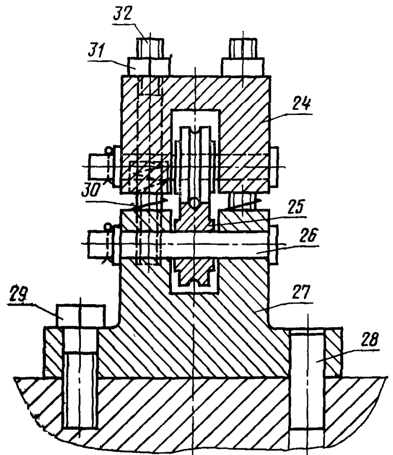
Г-Г повернуто
