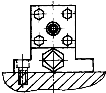
вид Д
