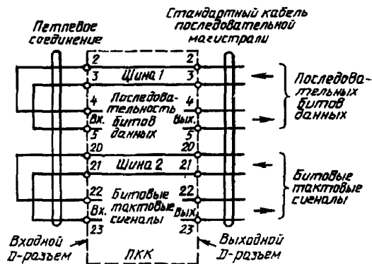
Пример использования контактов шин 1 и 2 D-соединителей
