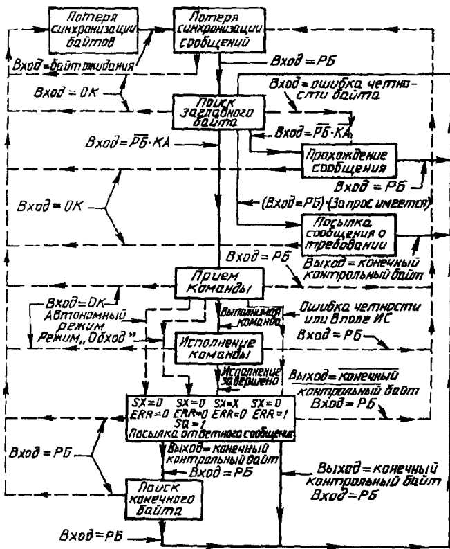
Последовательность основных состояний ПКК
