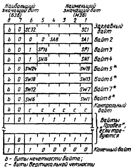
Командное сообщение: распределение битов
