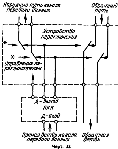
Пример переключения схемы для одного сигнала D-порта
