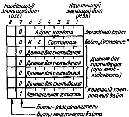
Ответное сообщение: распределение полей
