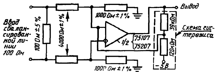
Пример приемника с гистерезисом, дополненным внешними резисторами
