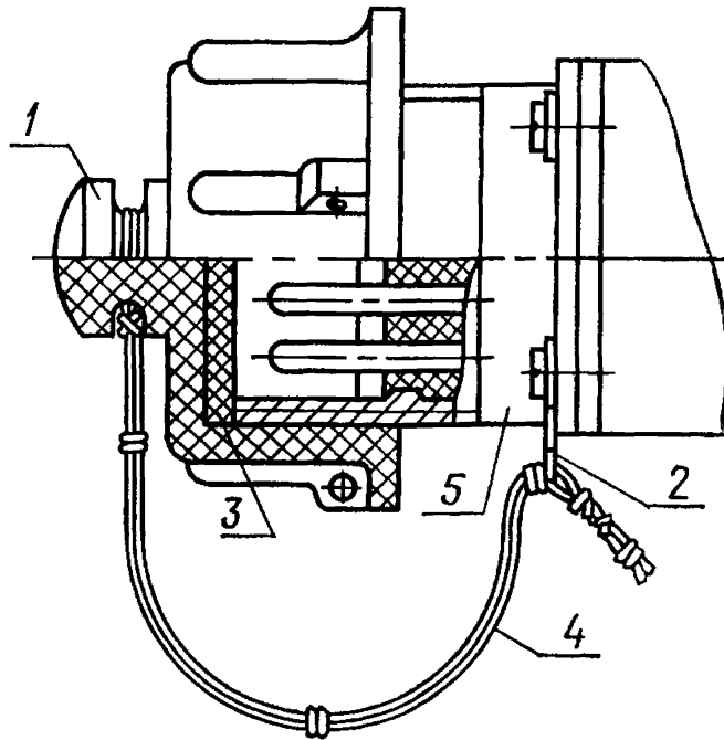
1 — крышка 1-М24×1; 2 — ушко 3,4, 3 — прокладка 10, марка резины 4 — капроновая нить ЗК l=300 j_s 17 ( \pm 2,6 ) мм, 5 — соединитель
