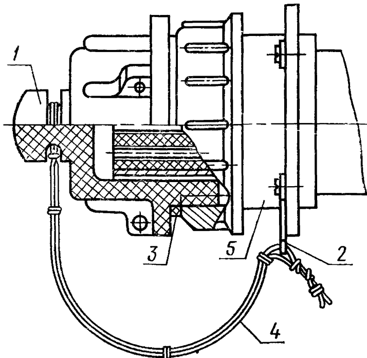
1 — крышка 2-М24×1—ЗД; 2 — ушко 3,4, 3 — прокладка 31, марка резины, 4 — леска 0,8 мм l=300 j_s 17 ( \pm 2,6 ) мм, 5 — соединитель
