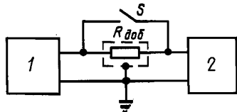
Схема определения входного сопротивления
