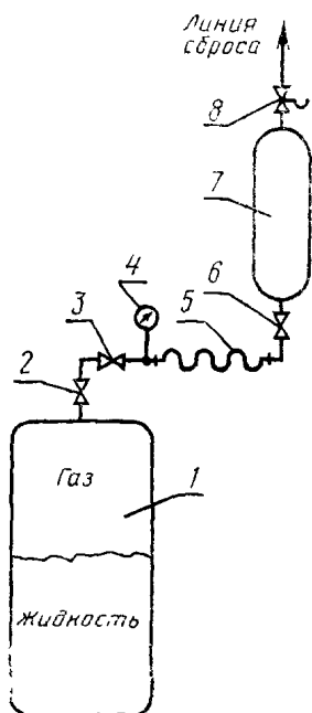
Схема отбора проб этилена и пропилена из газовой фазы
