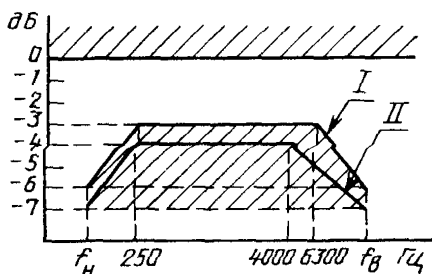
Допускаемая неравномерность амплитудно-частотной характеристики каналов воспроизведения и записи-воспроизведения
