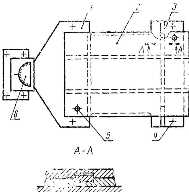
1 — плита; 2 — трафарет; 3 — шпонка; 4 — болт крепежный, 5 — штифт фиксирующий; 6 — узел точкой настройки
